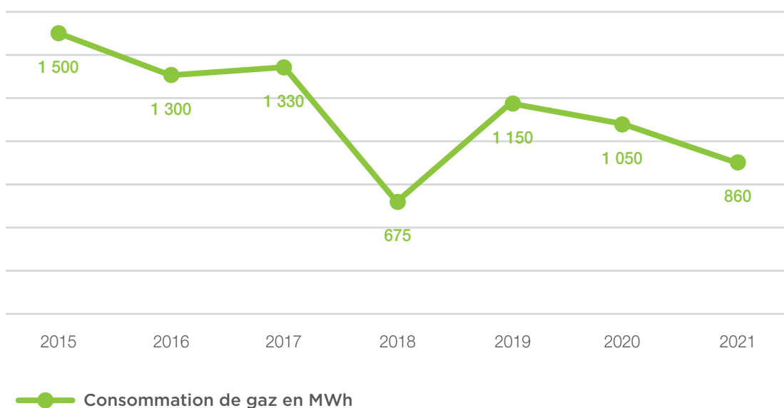
Évolution de la consommation de gaz en MWh 2015-2021
